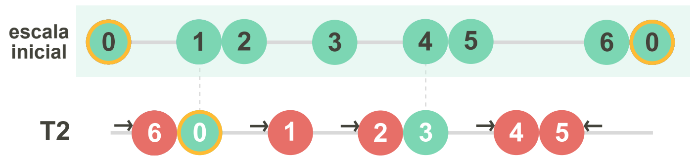
contraste = 5
