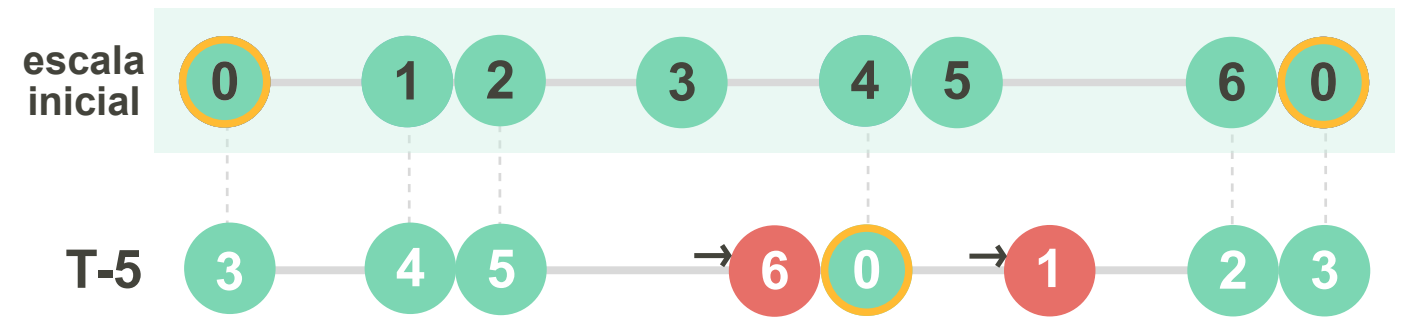
contraste = 2
