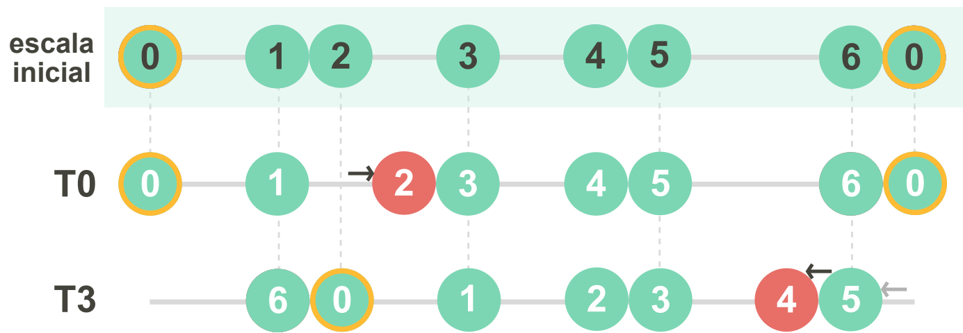
contraste = 1
