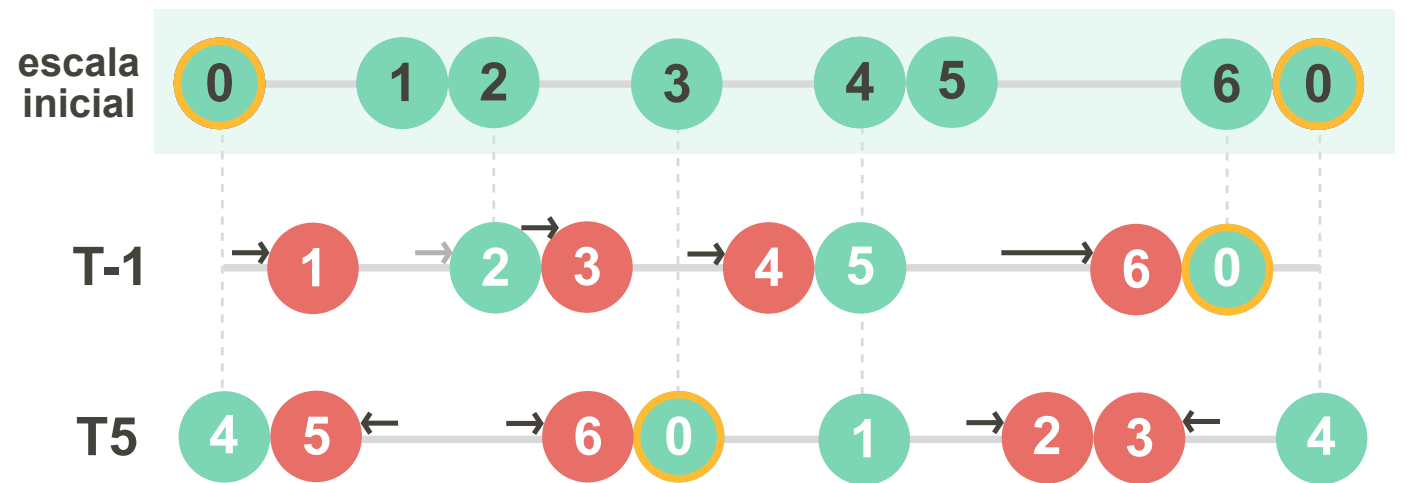
contraste = 4
