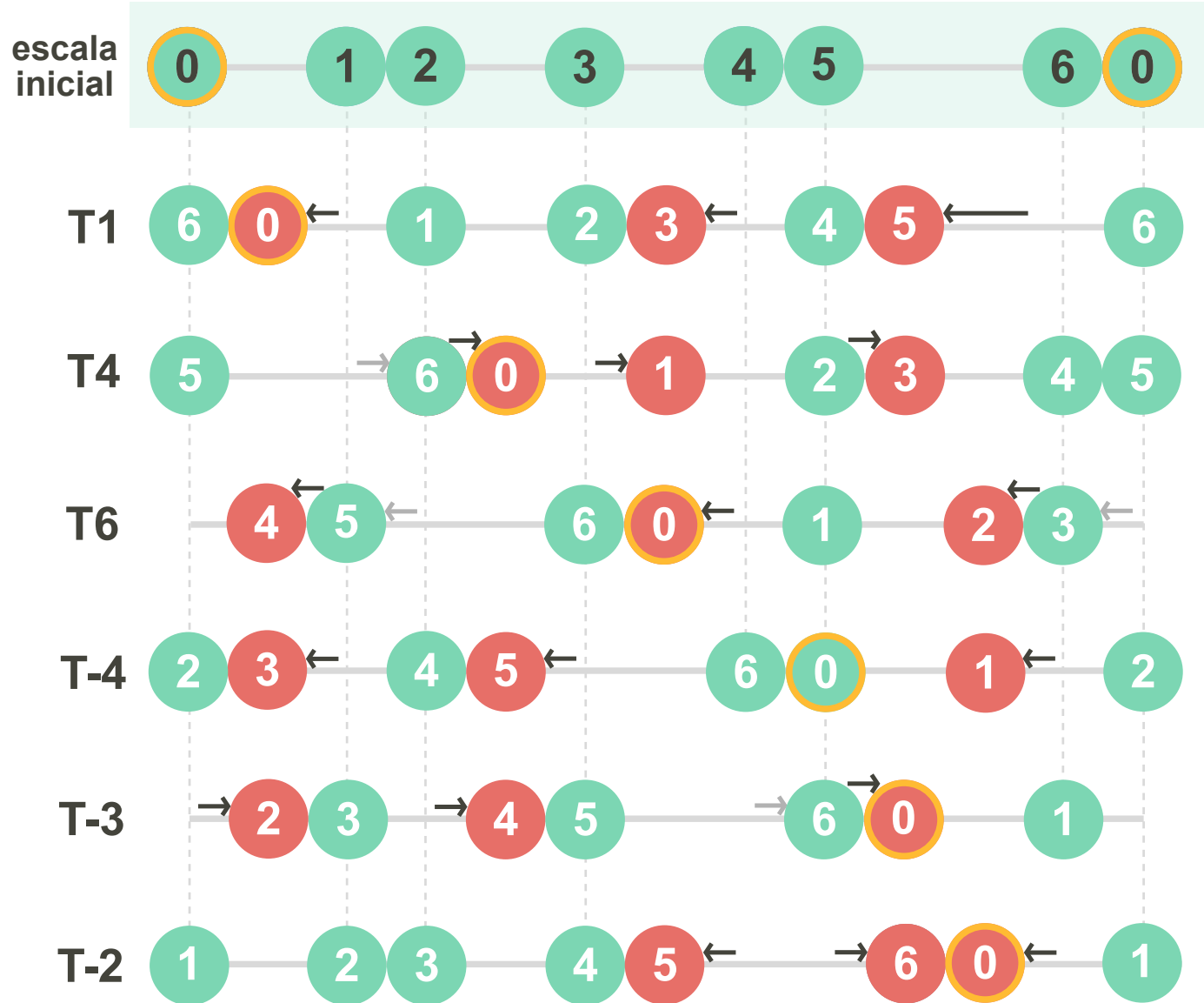
contraste = 3
